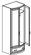
Шкаф для одежды 123b 2300x900x580
