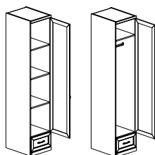
Шкаф для одежды 127ab 2300x450x580
